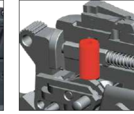
İğne kilidi
